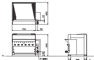
外形寸法(mm) : W700×D650×H640 Dimensions : W700×D650×H640
