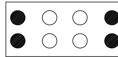
φ180二重バーナ インプット配置図
